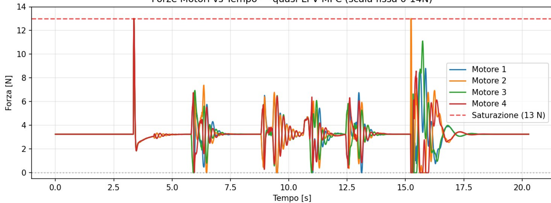
Forze Motori vs Tempo — quasi-LPV-MPC (scala fissa 0-14N)
